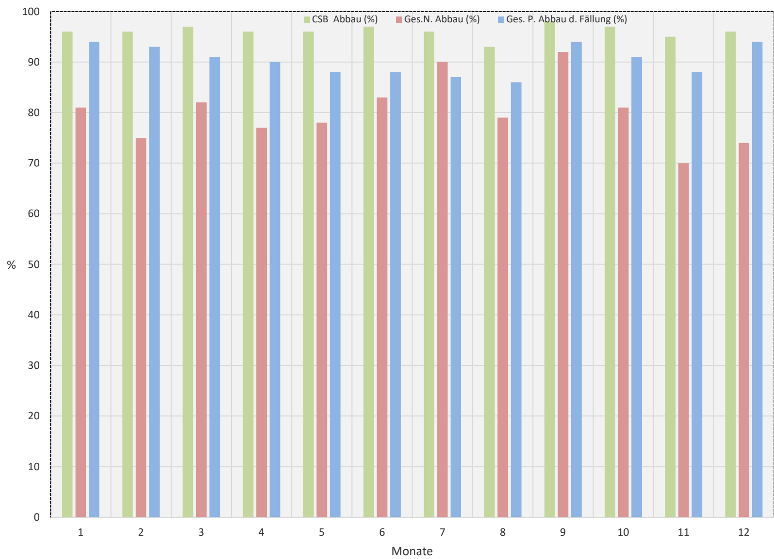
Kläranlage Gleisdorf 2023 - Reinigungsleistungen (%)
